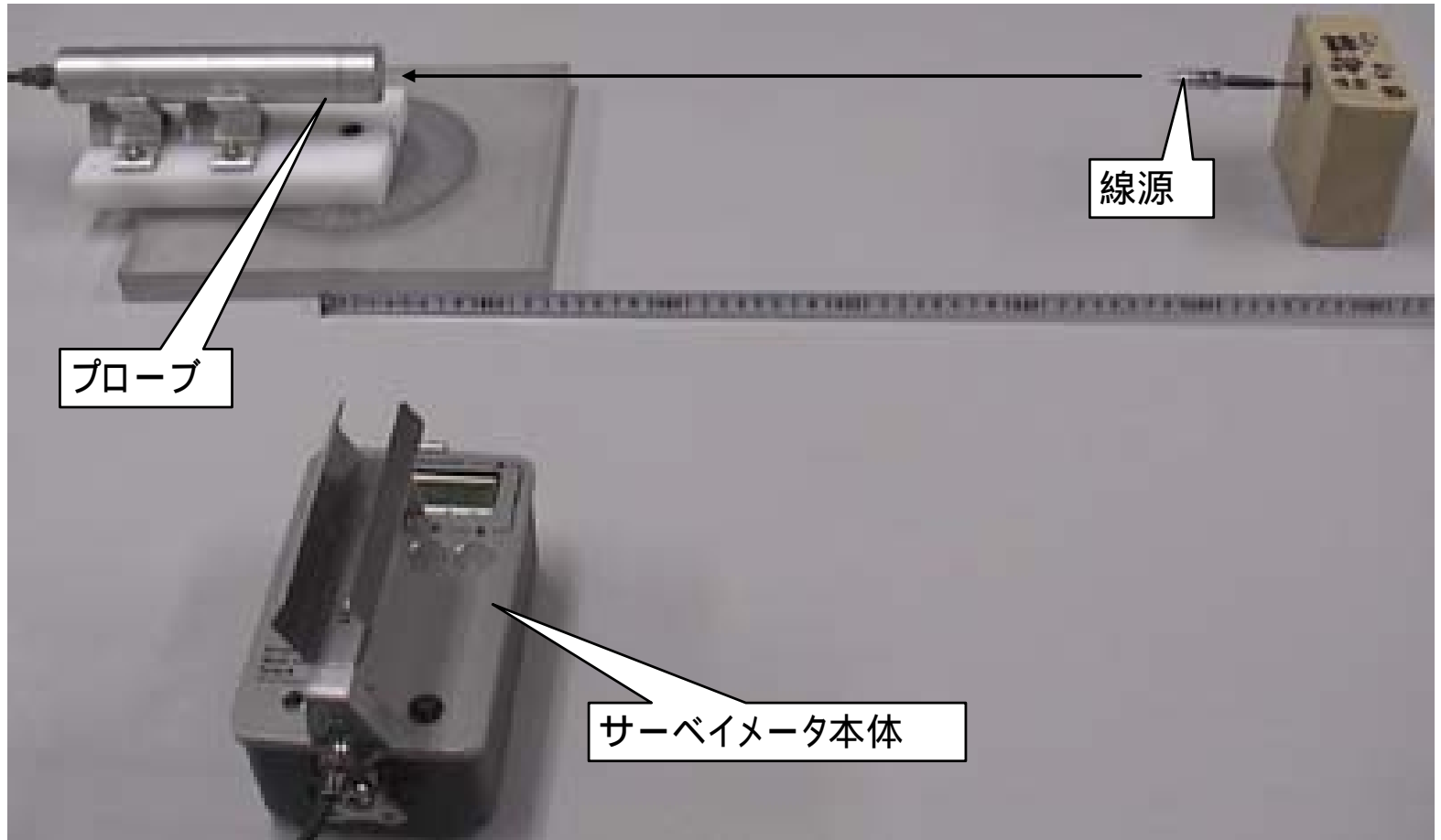
図10.16 方向依存性の測定配置写真
