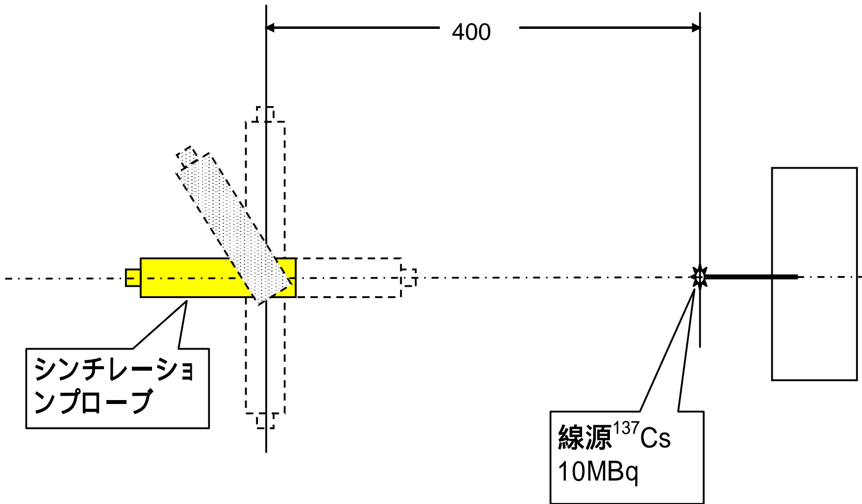
図10.17 方向依存性の測定配置図
